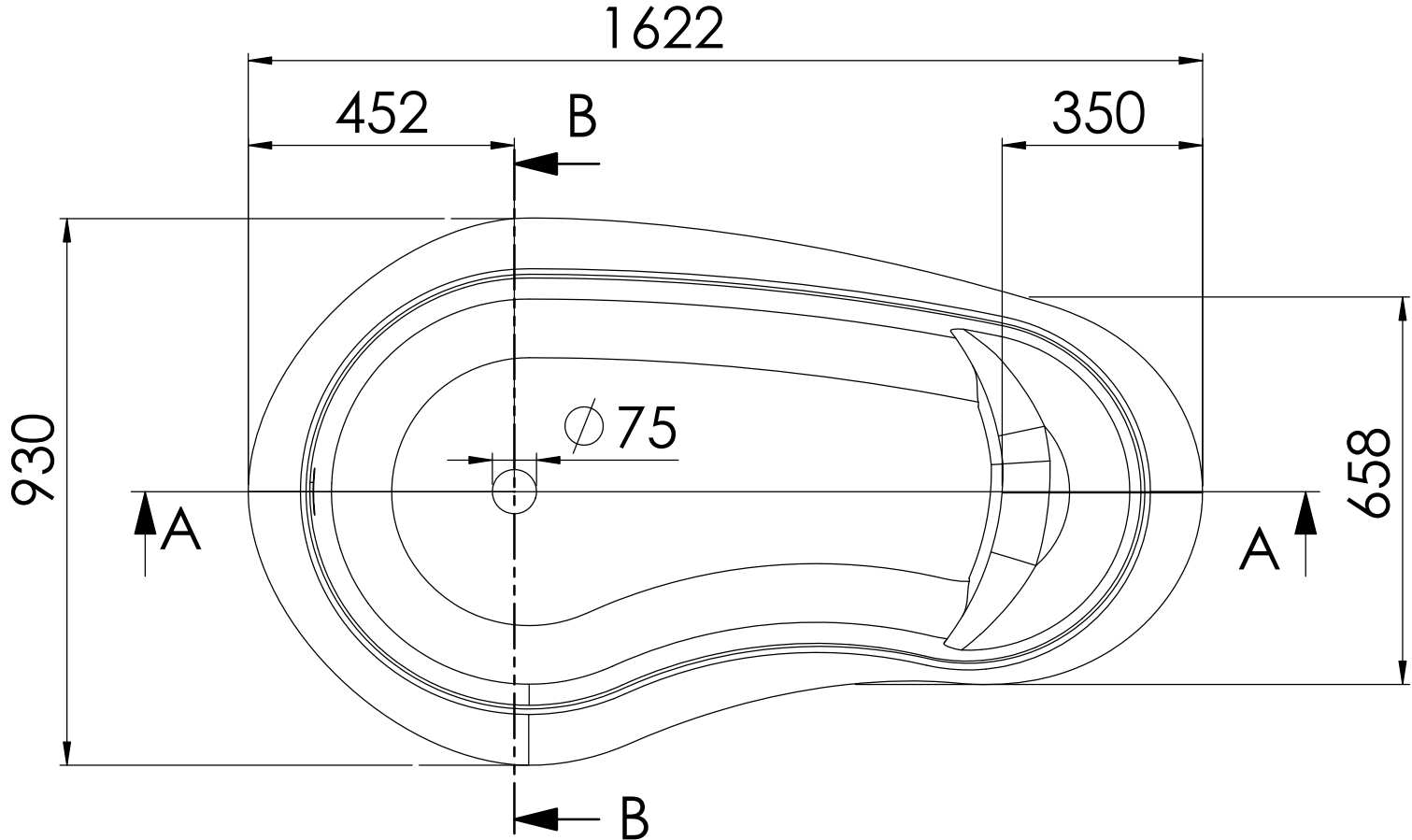
SCHNITT A-A
