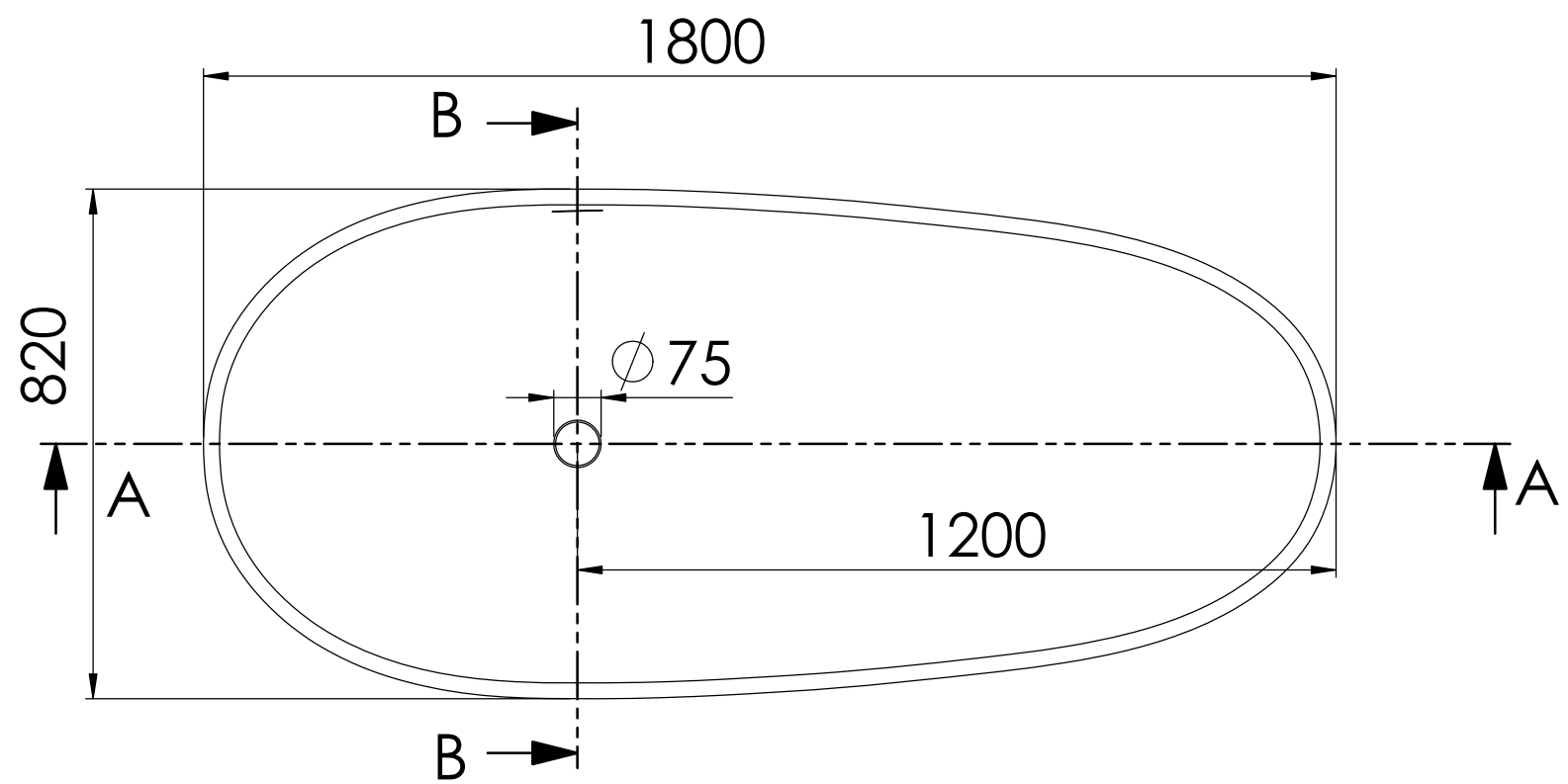
SCHNITT A-A
