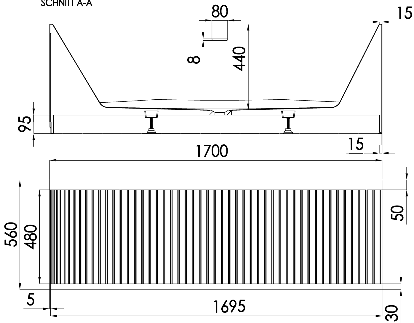
SCHNITT A-A
