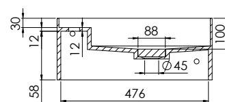
SCHNITT B-B
