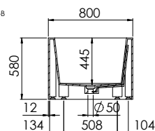
SCHNITT B-B
