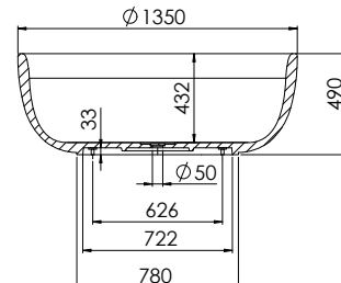
SCHNITT A-A
